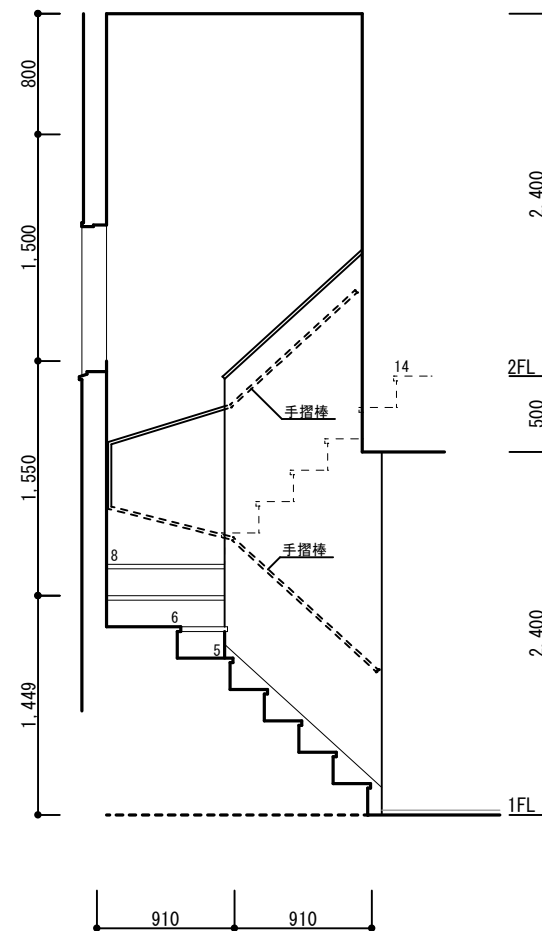
階段 断面図
